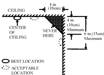
Figuur 3: Aanbevelingen om de rook & hitte detectoren op de best mogelijk locatie te installeren.
